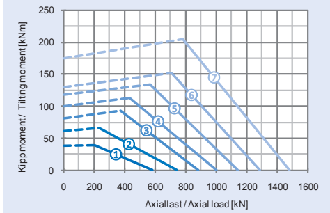
Schraubenkurve · Bolt Curve Laufbahnkurve · Raceway Curve
