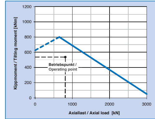
Grenzlastdiagramm · Limit load diagram
