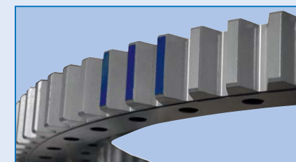
Kennzeichnung der Verzahnungseingstelle Marking of narrowest point of gear teeth
