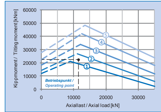
Grenzlastdiagramm (Beispiel) · Limit load curve diagram (example)
