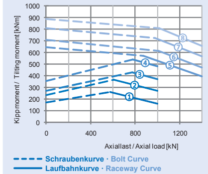
Grenzlastdiagramm · Statische Tragfähigkeit Limit load diagram · Static load capacity
