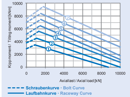
Grenzlastdiagramm · Statische Tragfähigkeit Limit load diagram · Static load capacity
