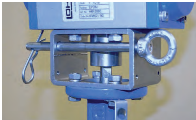
Arretierung unverriegelt
