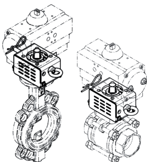
Arretierung unverriegelt
