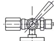
Zapfen / Spannmuffe mit Prüfflansch 60 x 25 mm DIN 16 263
