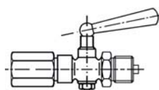
Zapfen / lose Mutter mit Prüfflansch 60 x 25 mm mit Stopfbuchse
