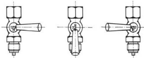
Ausblasestellung Zuleitung offen Druckmessgerät außer Betrieb Messstoff entweicht ins Freie
