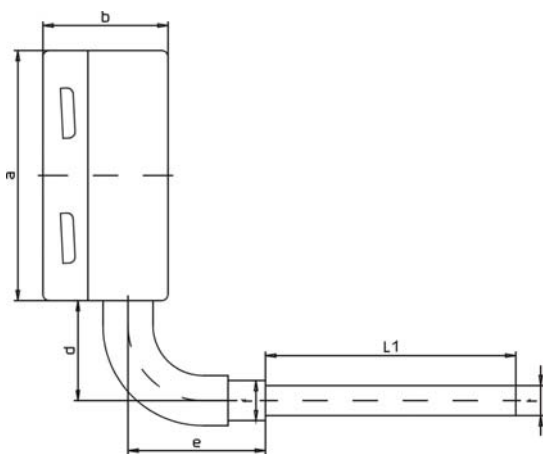
Anschluss in Winkelform
