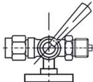
Zapfen / lose Mutter mit Prüfflansch 60 x 25 mm mit Stopfbuchse
