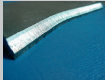
Coupe chanfrein avec talon (coupe-Y) Taglio a smusso ad Y
